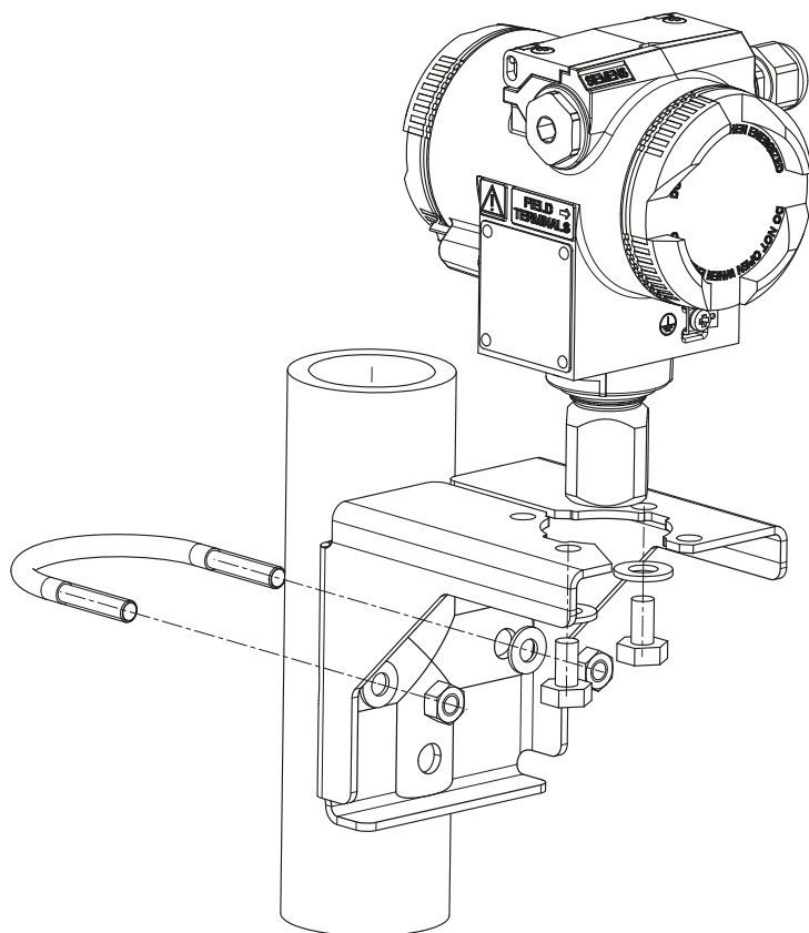
Bild 3-1 Befestigung des Messumformers mit Montagewinkel
