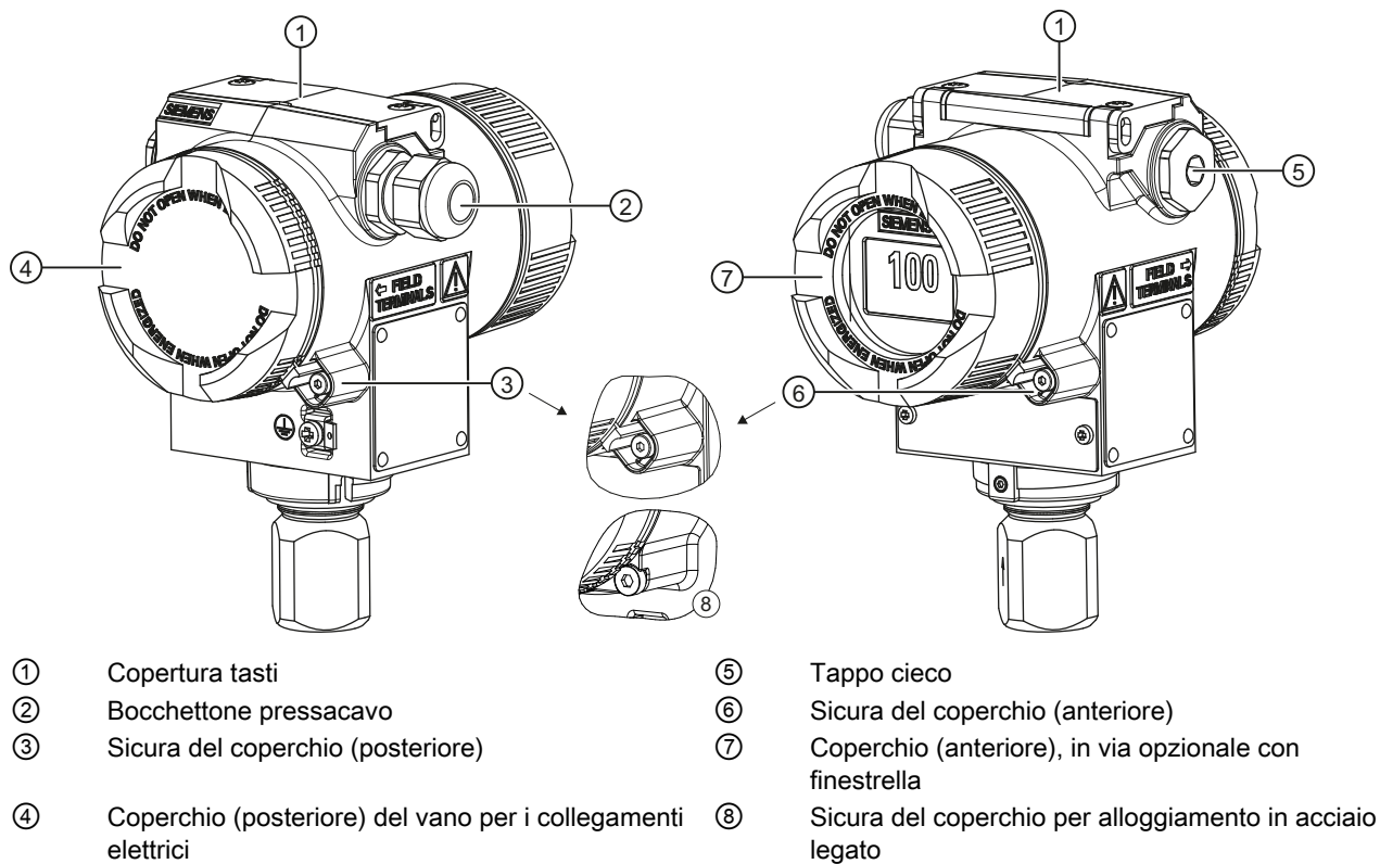
Figura 4-1 Vista del trasmettitore di misura. A sinistra: vista posteriore; a destra: vista anteriore
