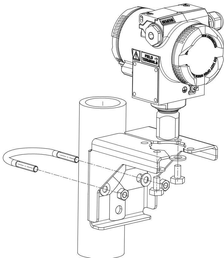
Figura 3-1 Fijación del transmisor con escuadra
