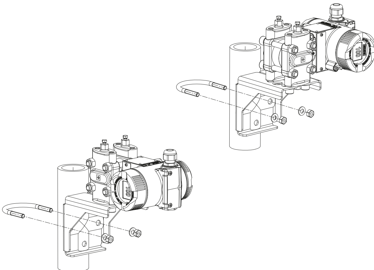
Figura 3-3 Fissaggio con angolare, nell'esempio pressione differenziale con condutture pressione effettiva verticali
