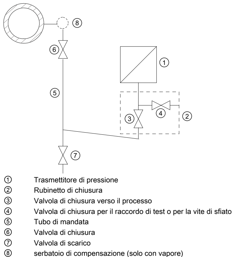
Figura 5-1 Misurazione del vapore
