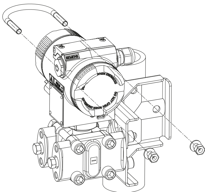
Figura 3-2 Fijación del transmisor con escuadra en el ejemplo de presión diferencial con tuberías horizontales de presión efectiva
