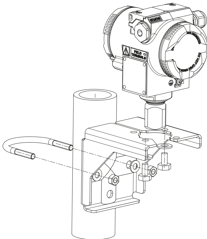
Figura 3-1 Fissaggio del trasmettitore con angolare
