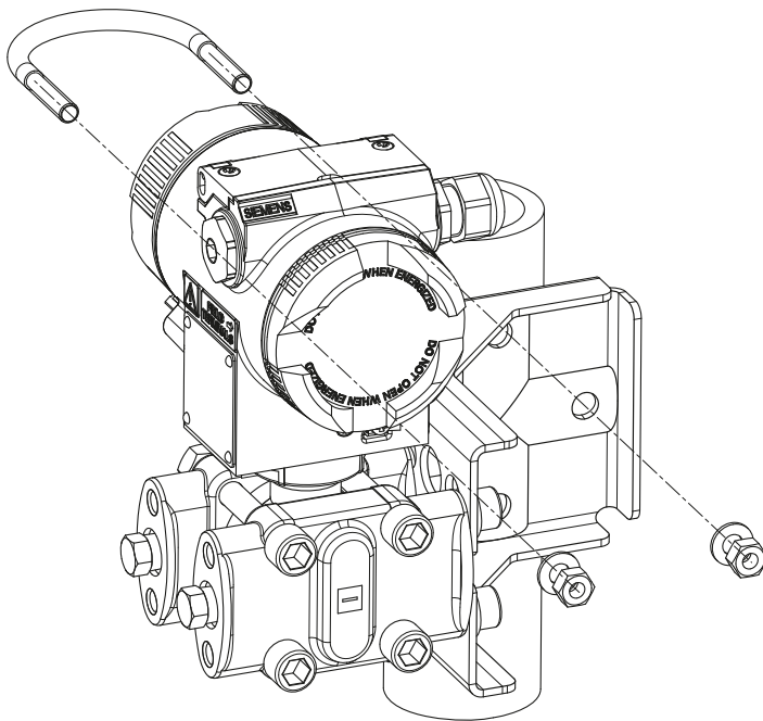
Bild 3-2 Befestigung des Messumformers mit Montagewinkel am Beispiel Differenzdruck bei waagrechten Wirkdruckleitungen
