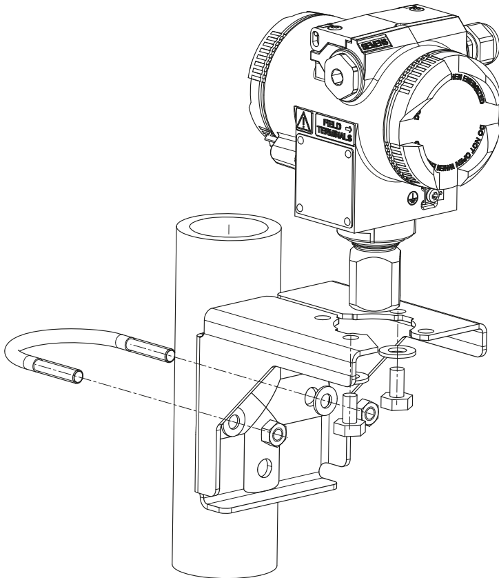
Figure 3-1 Fixation du transmetteur de mesure avec l'équerre de montage
