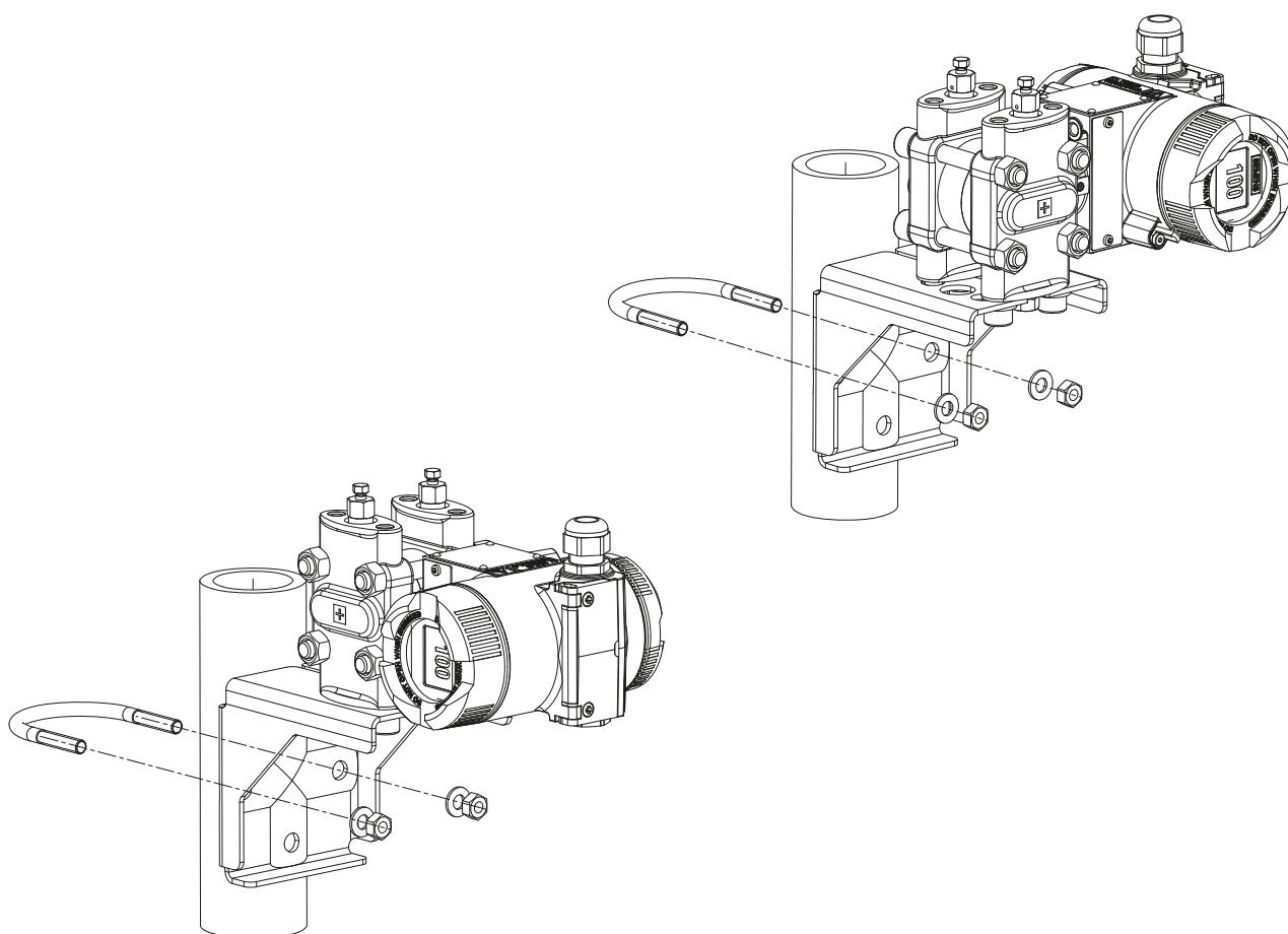
Figure 3-3 Fixation avec l'équerre de montage à l'exemple de la pression différentielle sur des conduites de pression active verticales
