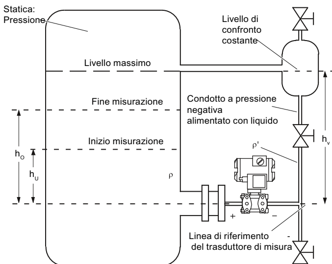
Schema di misura a contenitore chiuso (forte condensa)
