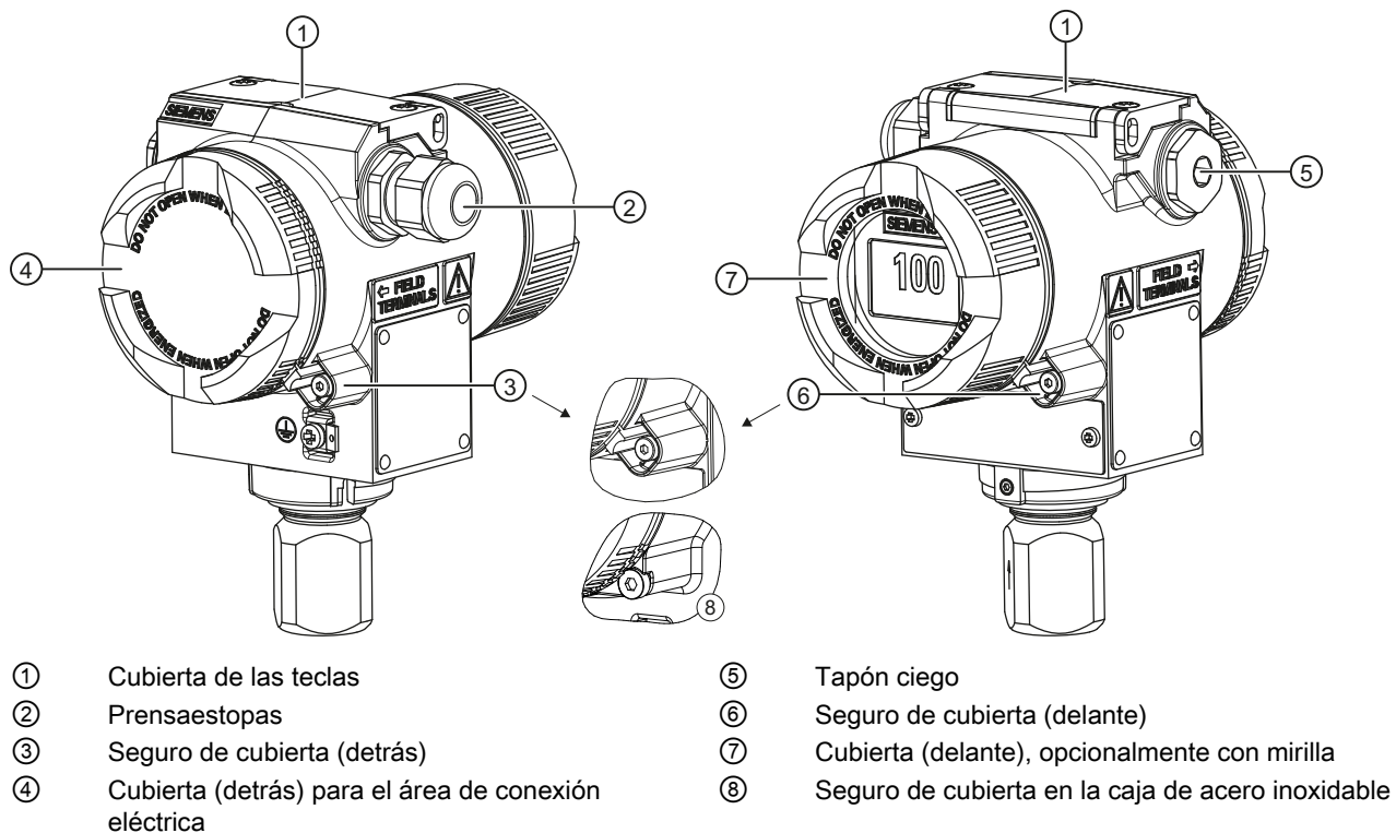
Figura 4-1 Vista del transmisor: Izquierda: Vista posterior, derecha: Vista frontal
