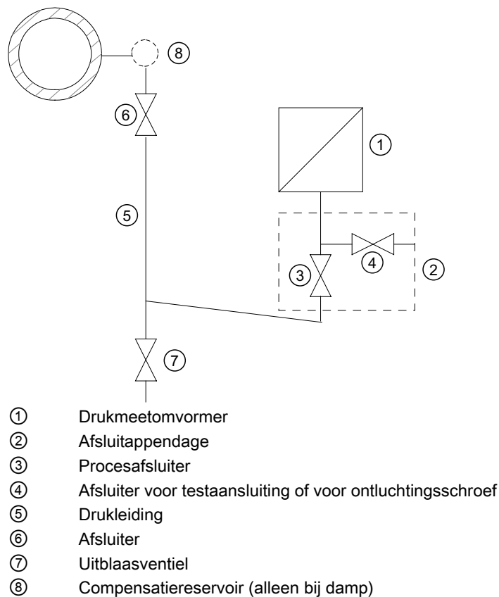
Beeld 5-1 Meten van damp
