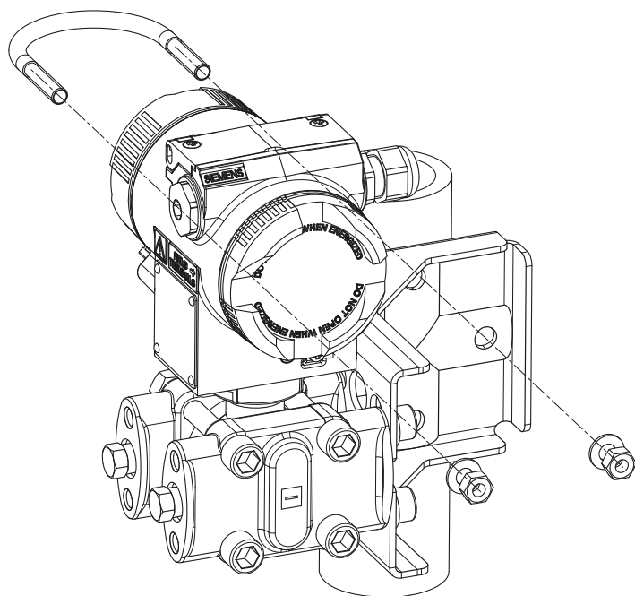
Figura 3-2 Fissaggio del trasmettitore con angolare, nell'esempio pressione differenziale con condutture pressione effettiva orizzontali
