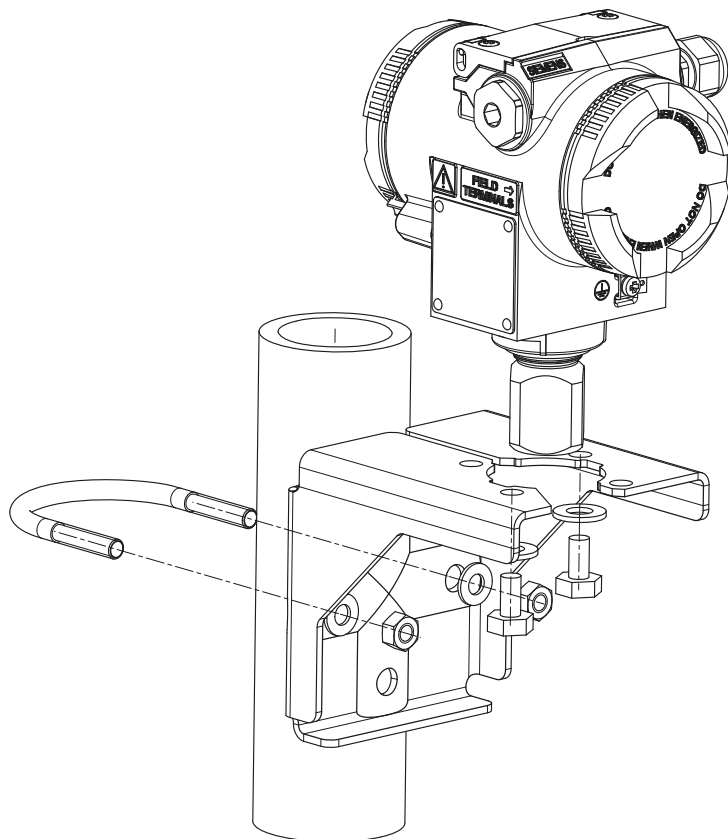
Beeld 3-1 Bevestiging van de meetomvormer met montagehoek
