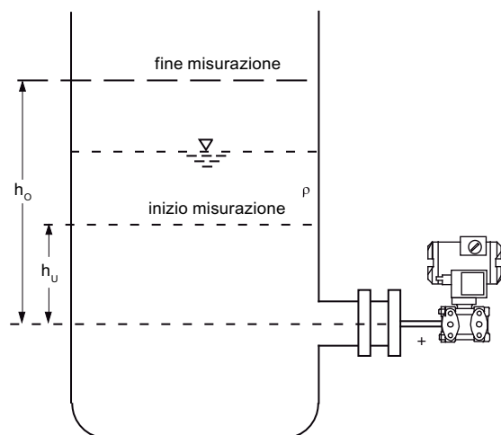
Schema di misura a contenitore aperto
